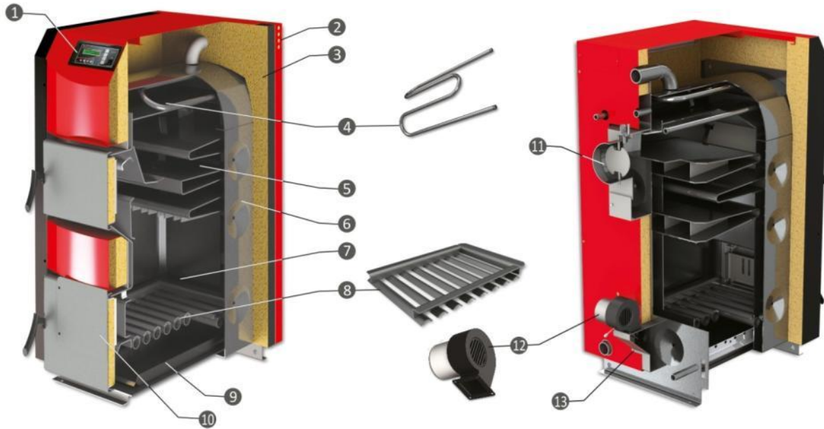
Диаграмма 10. Элементы Котла WBS Active
