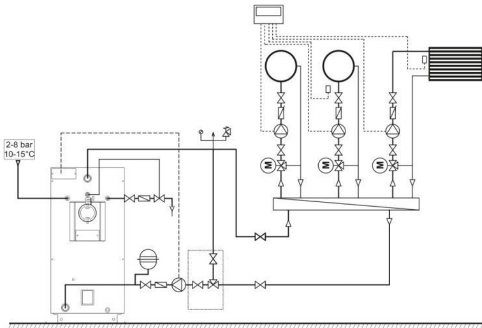
Диаграмма 6. Соединение BURNiT WBS Active котла к 3-х ходовому ветилю
