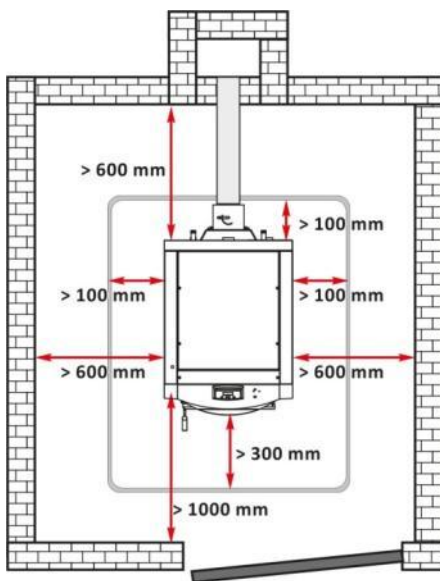
Диаграмма 1 Рекомендуемые расстояния между котлом и стенами.
