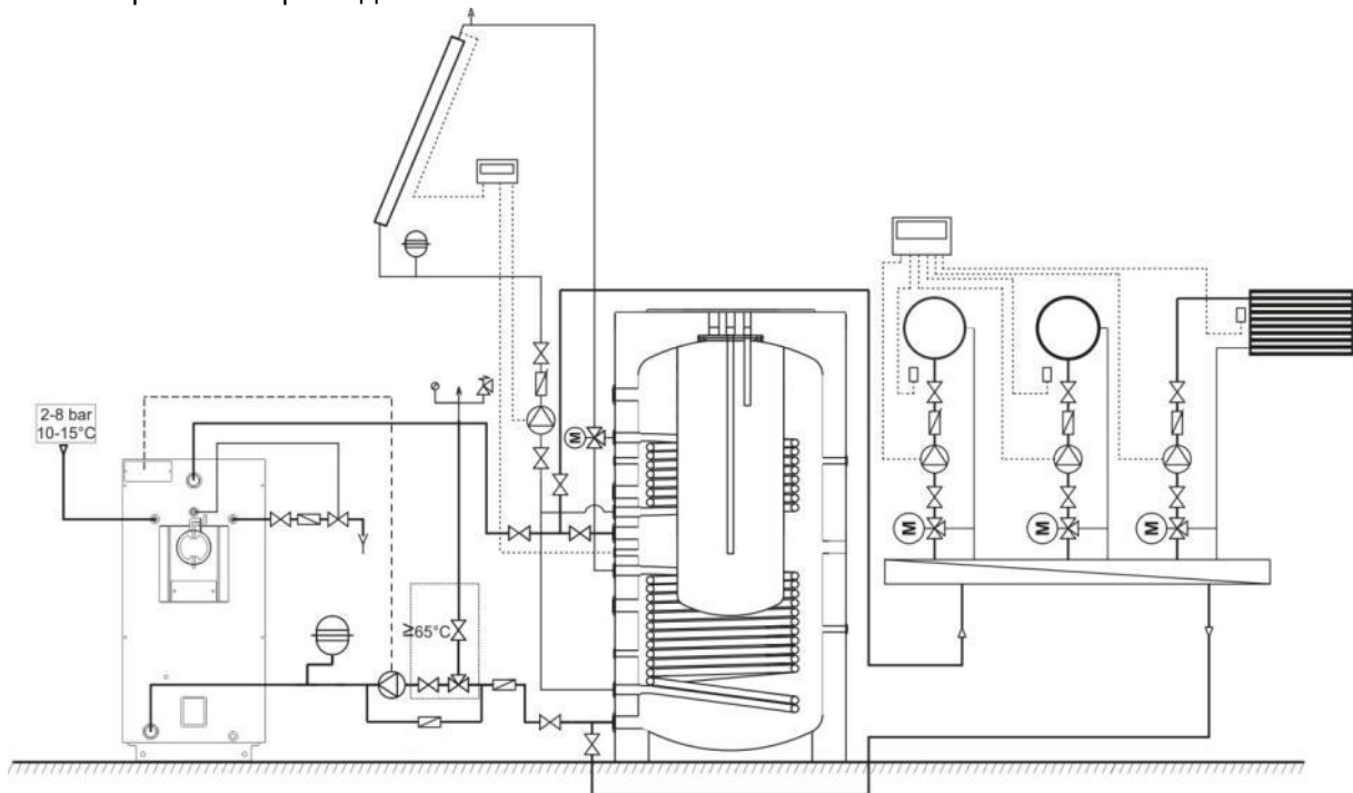
Диаграмма 8. Соединение BURNiT WBS Active котла с комбинированным баком KSC2, плоским коллектором ПК и трехходовым клапаном
