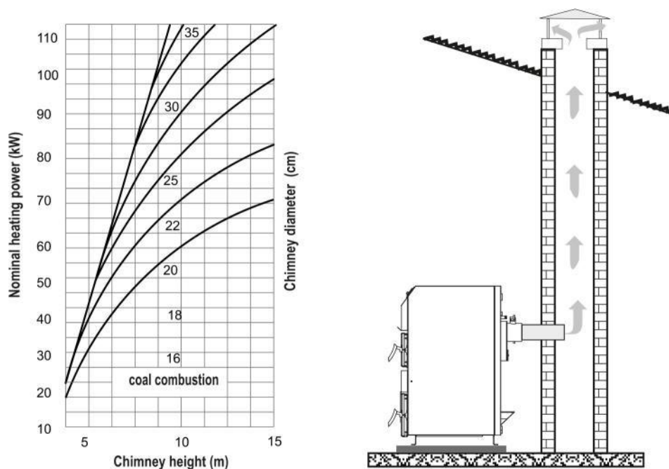
Диаграмма 4. Размер котла и параметры дымохода
